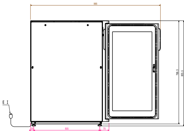
Boven aanzicht
